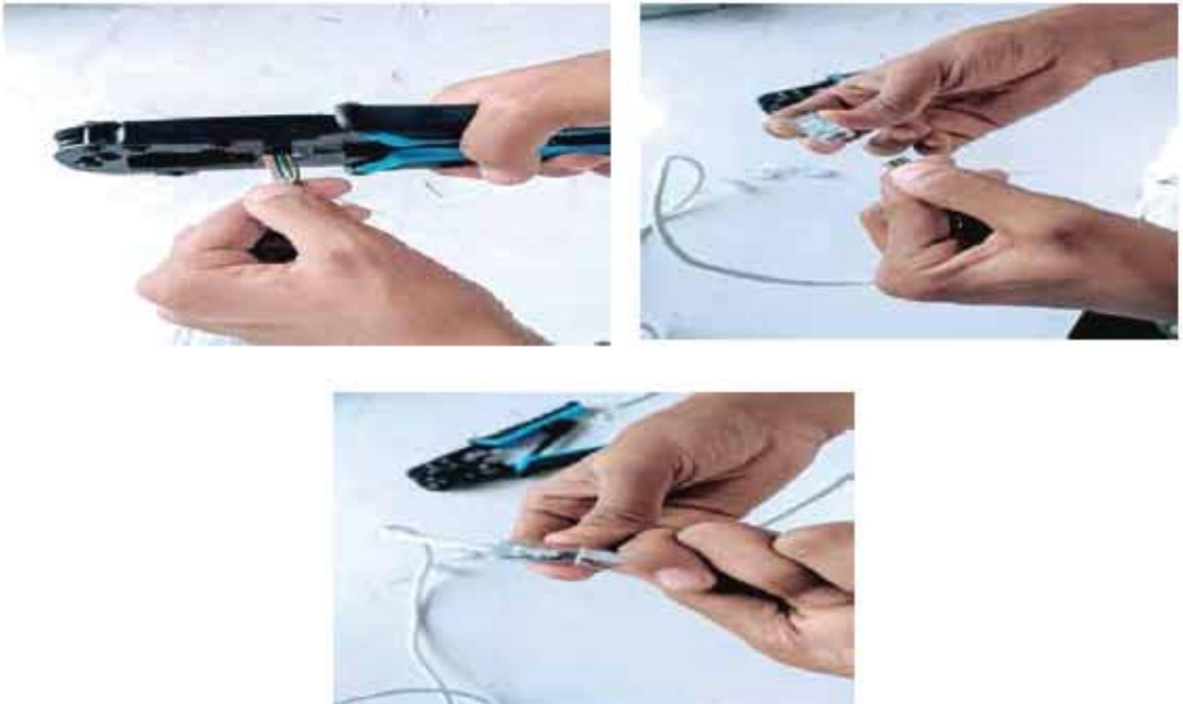
চিত্র-১.৪২ চিকন তারগুলো আরজে-৪৫ কানেক্টর এর মধ্যে ঢুকানোর দৃশ্য।
