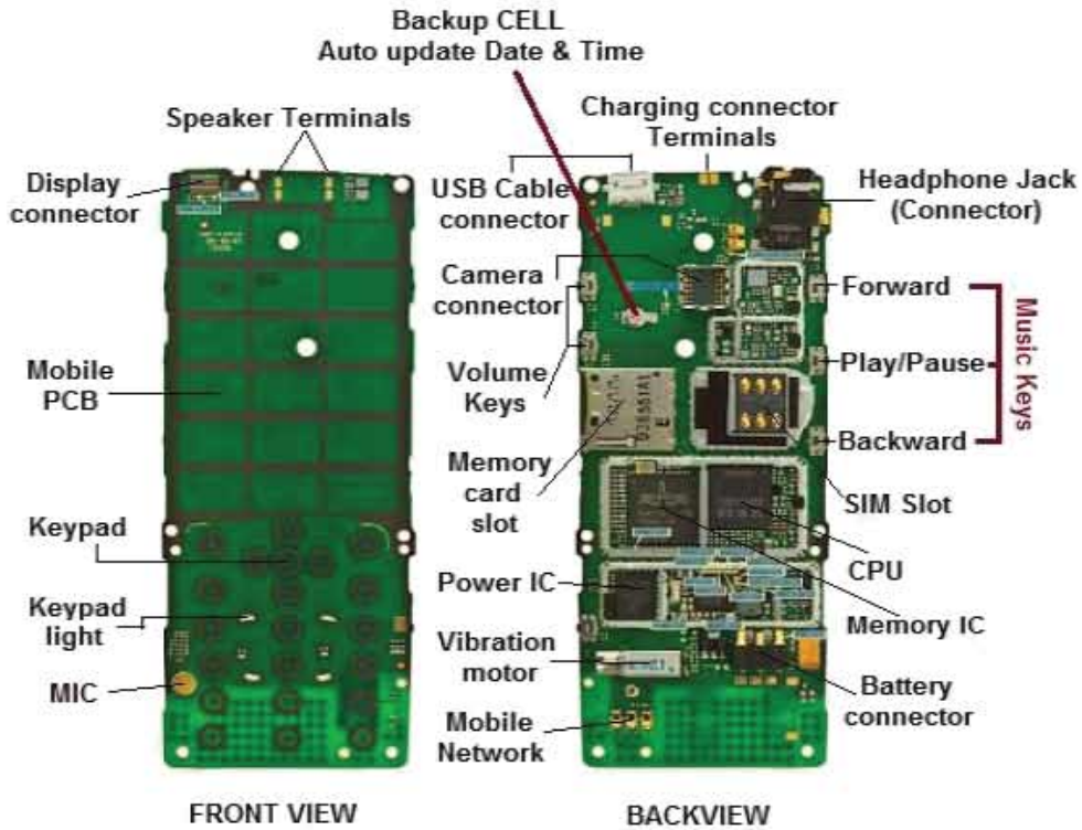
চিত্র-১.৪ একটি সাধারণ জিএসএম মোবাইল ফোনের আভ্যন্তরীণ বিভিন্ন (সামনের ও পিছনের দৃশ্য সমূহ) অংশসমূহ
