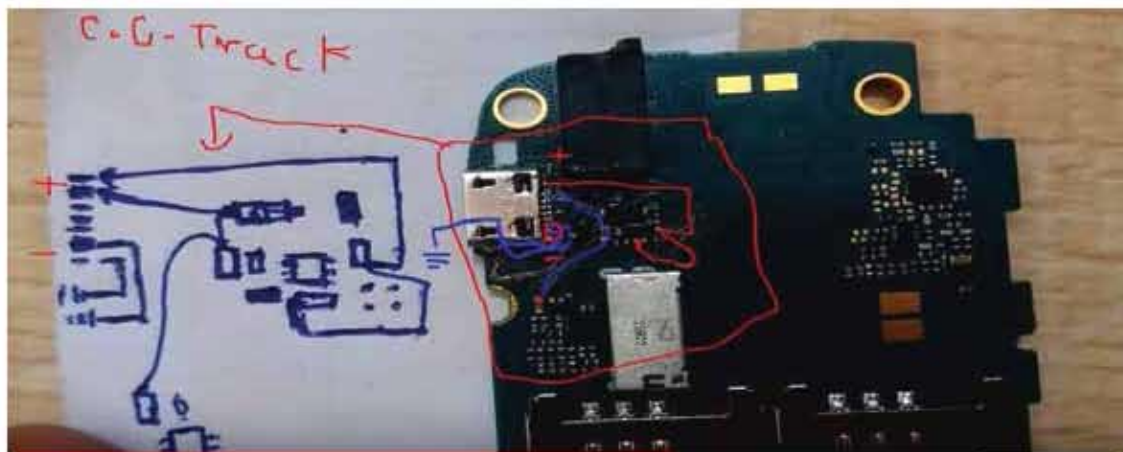
চিত্র- চার্জিং সেকশন এর ভারখাম (Mobile Phone Model: SAMSUNG METRO 313, 310)
