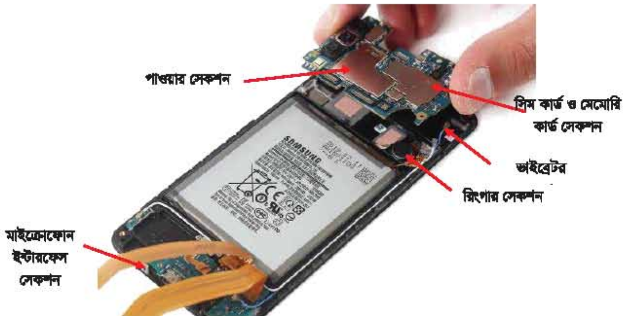
চিত্র - ৪.৩ স্মার্ট মোবাইল ফোনের বিভিন্ন সেকশন (Mobile Phone Model: Samsung Galaxy A50)
