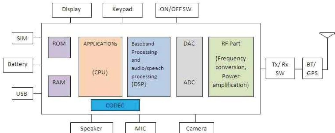
চিত্র-৩.৫ ফিচার মোবাইল ফোনের ব্লক ডায়াগ্রাম
