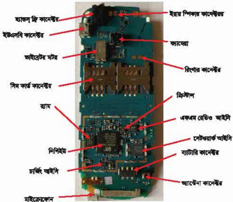
চিত্র-৩.২০ কিচর মোবাইল ফোনের বিভিন্ন কম্পোনেন্ট
