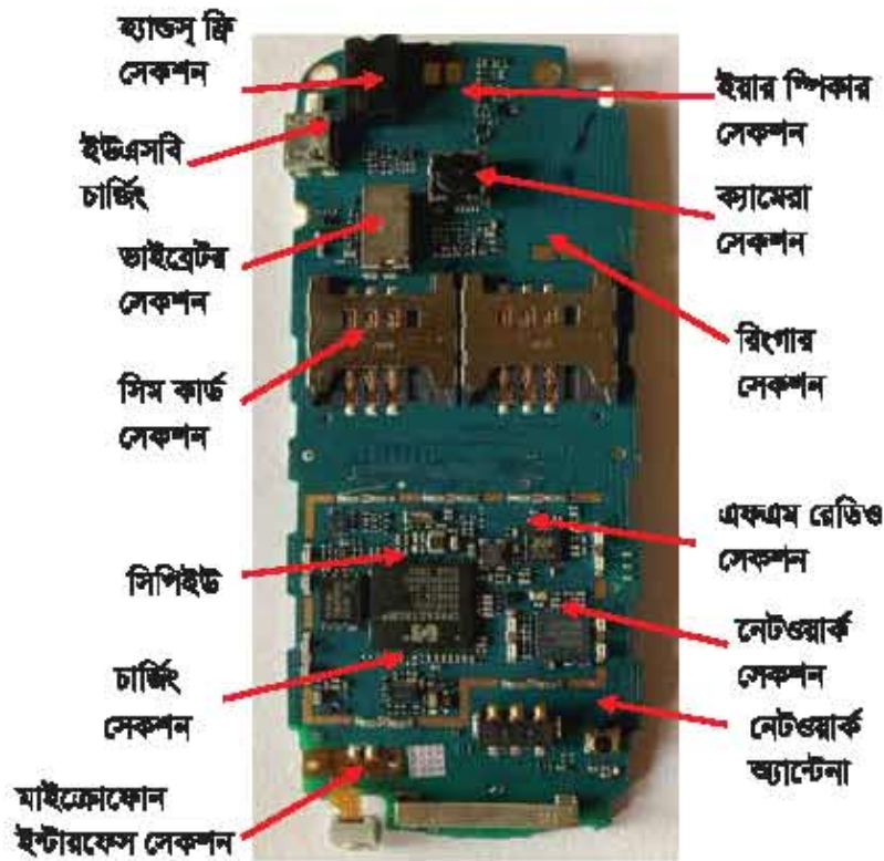
চিত্র-৩.৪ ফিচার মোবাইল ফোনের বিভিন্ন সেকশন
