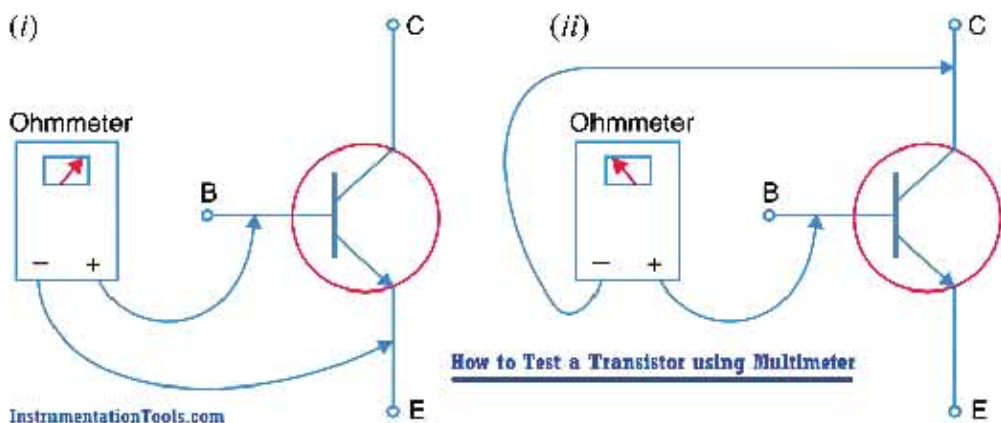
চিত্র-১.১০০ অ্যানালগ মাল্টিমিটার দিয়ে ট্রানজিস্টর পরীক্ষাকরণ
