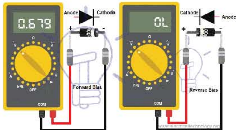
চিত্র-১.৯৯ ডিজিটাল বাস্টিমিটার দিয়ে ডায়োড পরীক্ষাকরণ
