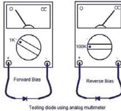
চিত্র-১.৯৮ অ্যানালগ বাস্টিমিটার দিয়ে ডায়োড পরীক্ষাকরণ
