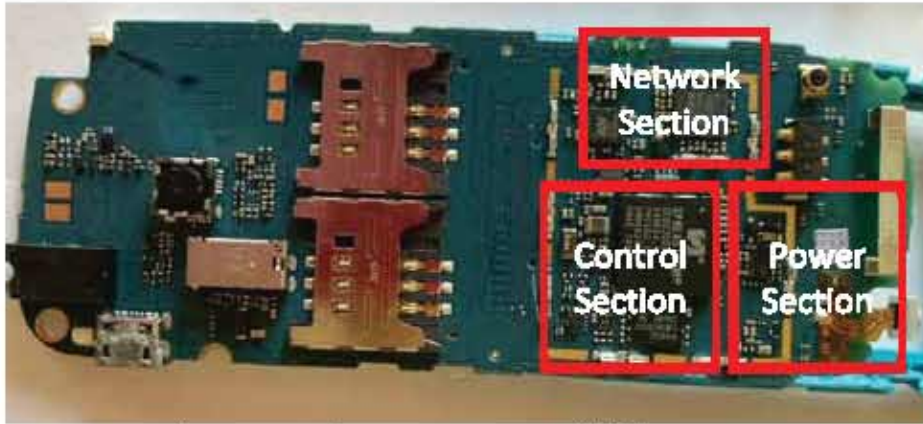
চিত্র-২.৩ মোবাইল ফোনের মাদার বোর্ডের বিভিন্ন সেকশন
