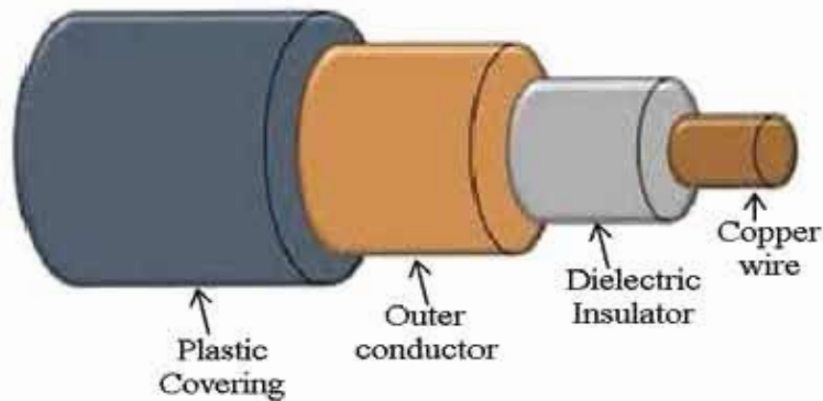
চিত্র- ১.৩৭ কো- অক্সিয়াল কেবুল
